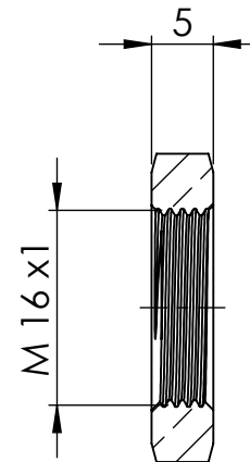
Ansicht / view A-A
